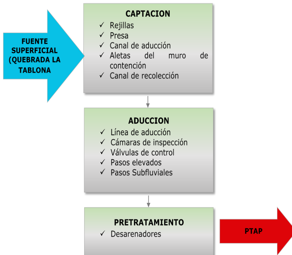
Grafico 2. Diagrama de bloques operación de tratamiento fuente superficial.
