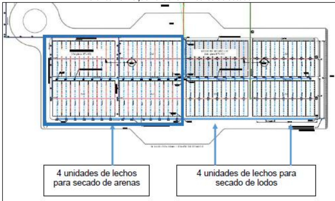
Grafico 13. Esquema General Lechos de secado
