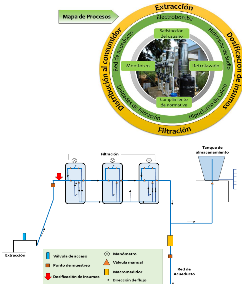
Grafico 27. Diagrama de flujo - Sistemas de Tratamiento de captación subterránea Baja Producción.
