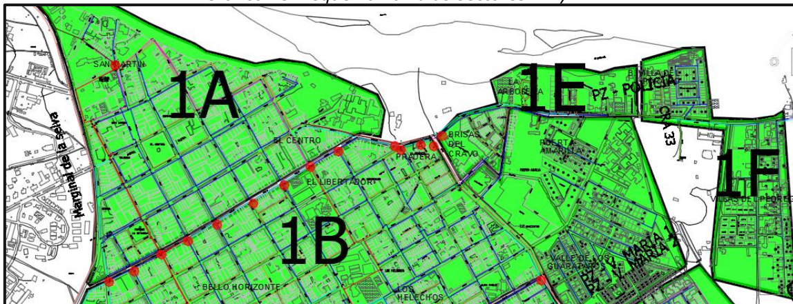
Grafico 23. Esquema válvulas sectores 1A y 1B
