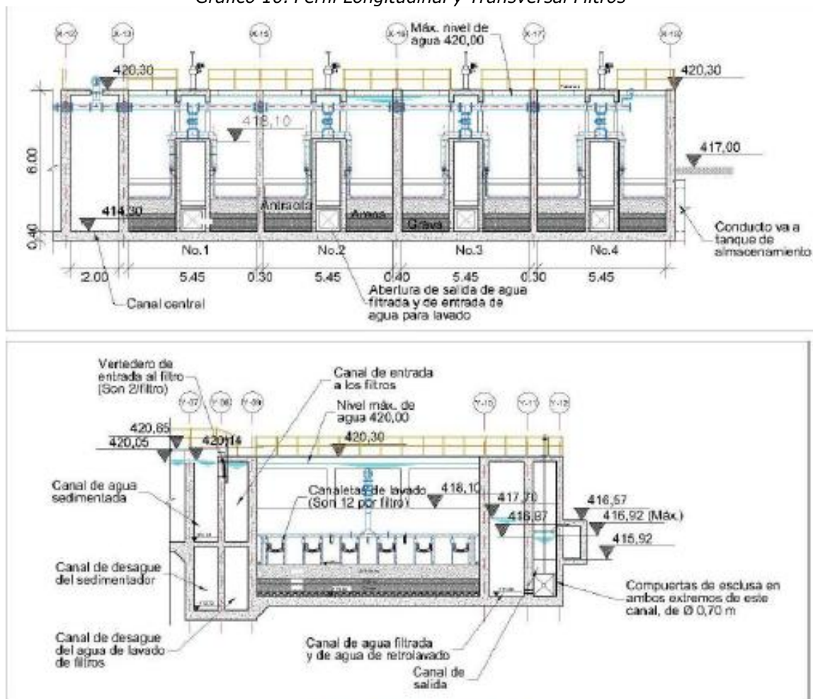
Grafico 10. Perfil Longitudinal y Transversal Filtros
