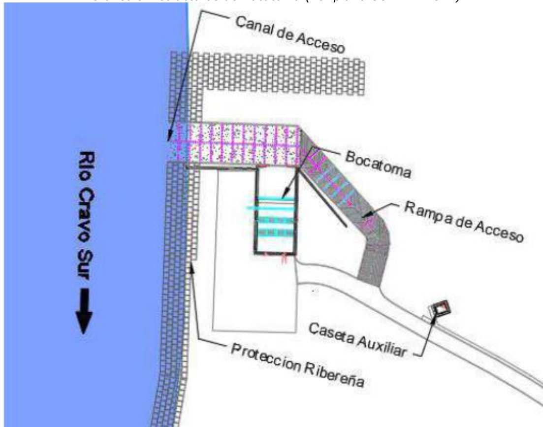
Grafico 3. Estructuras de Bocatoma (ver plano CGE-R 21 CAY)
