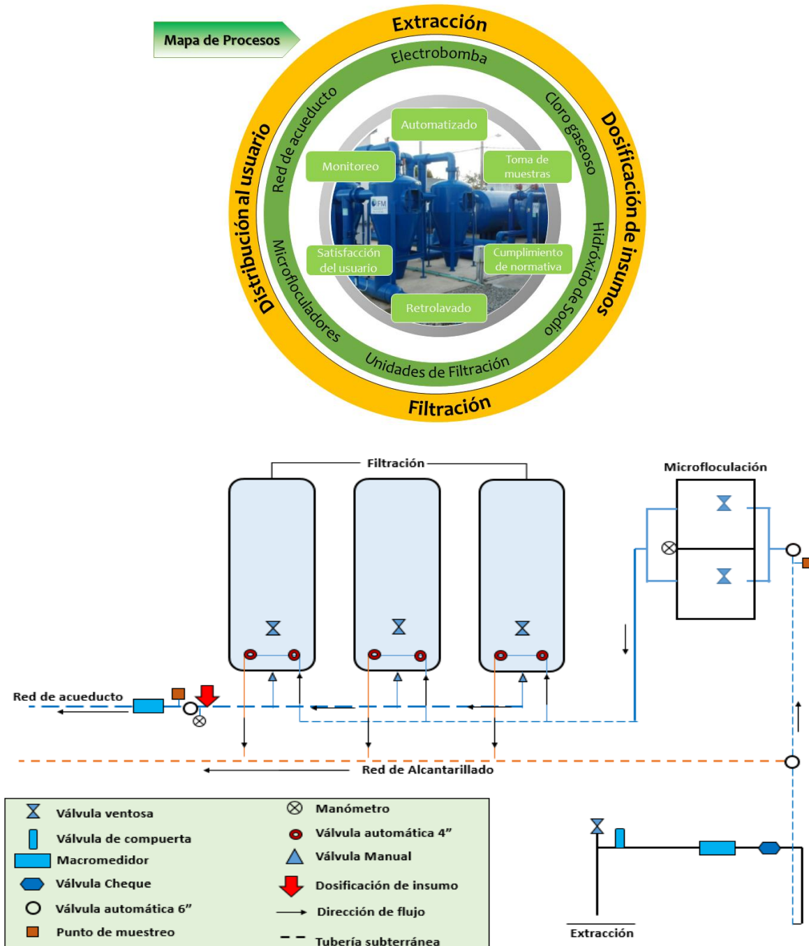
Grafico 26. Diagrama de flujo - Sistemas de Tratamiento de captación subterránea Gran Producción.
