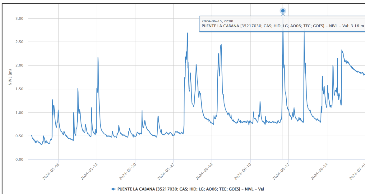
Grafico 37. Niveles altos, rio Cravo Mes de Julio 2024
