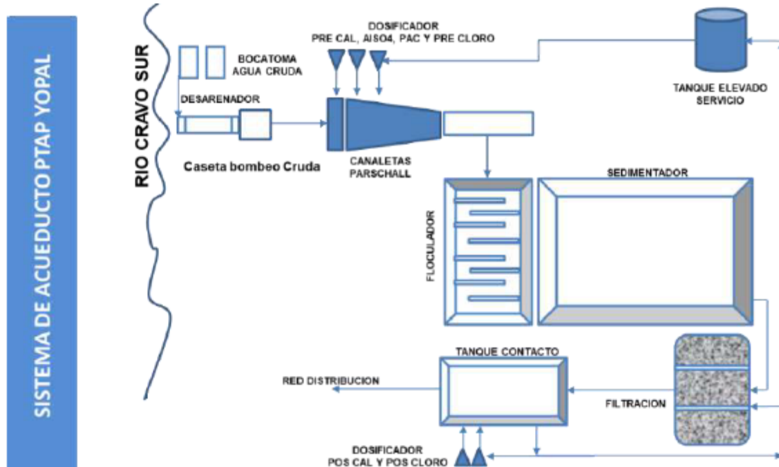
Grafico 5. Esquema Procesos PTAP Yopal
