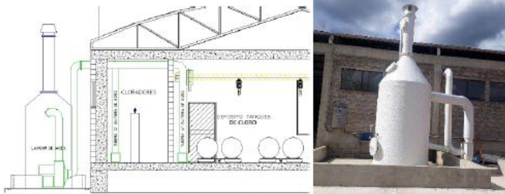
Grafico 11. Sistema de Neutralizacion de Fugas de Cloro Scrubber
