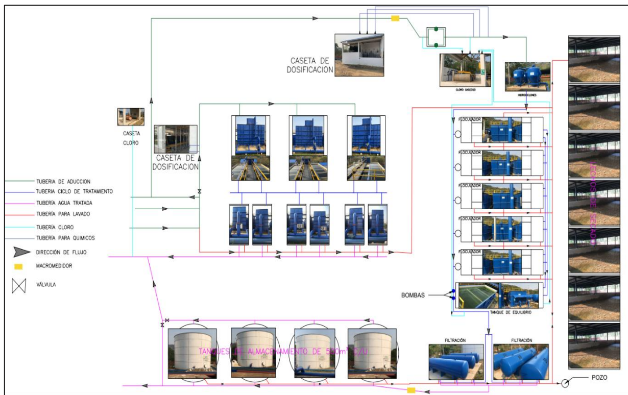
Grafico 18. Diagrama de flujo - Sistema Alterno de Tratamiento de Agua Potable.
