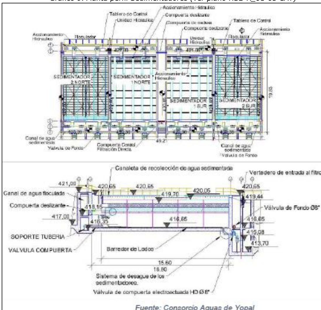
Grafico 9. Planta perfil Sedimentadores (ver plano HSE-R_01-03 CAY)
