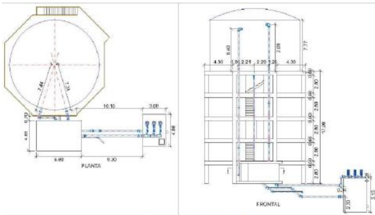
Grafico 12. Tanque de Servicio (ner planos HTS-R _01-04 CAY)
