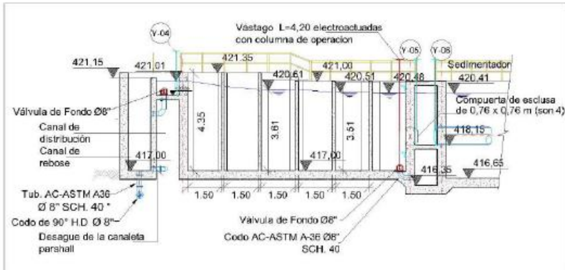
Grafico 8. Compuertas Floculadores (ver planos HFL-R 01-02 CAY)
