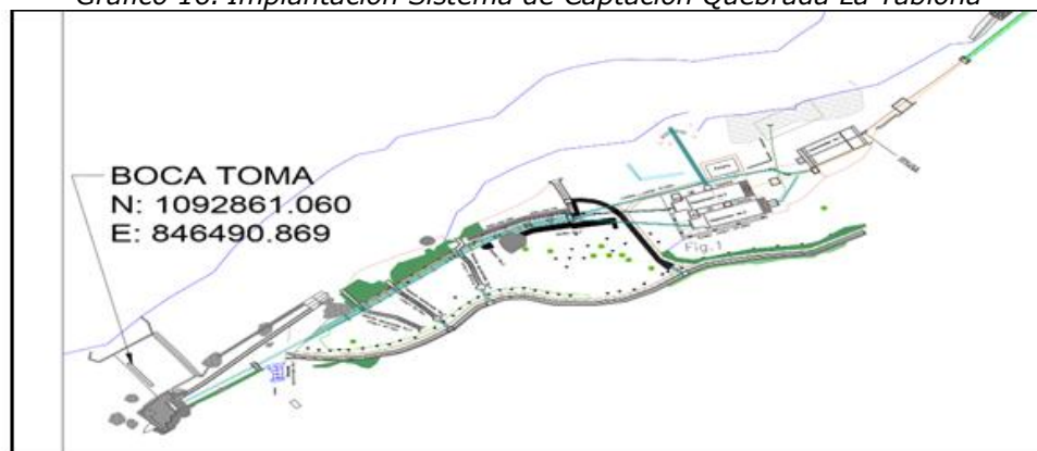
Grafico 16. Implantación Sistema de Captación Quebrada La Tablona
