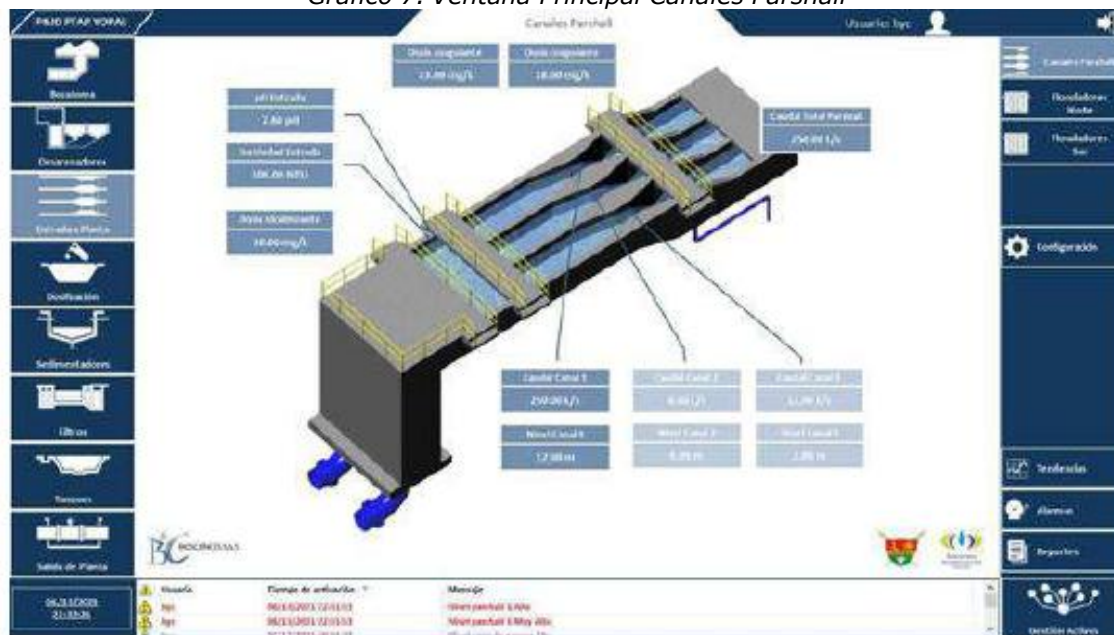
Grafico 7. Ventana Principal Canales Parshall
