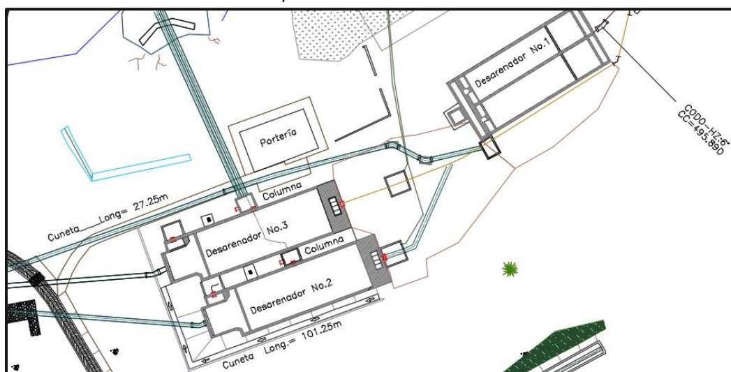
Grafico 17. Implantación Desarenadores la Tablona
