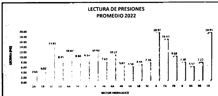
Gráfica. Presiones del servicio por sector hidráulico
